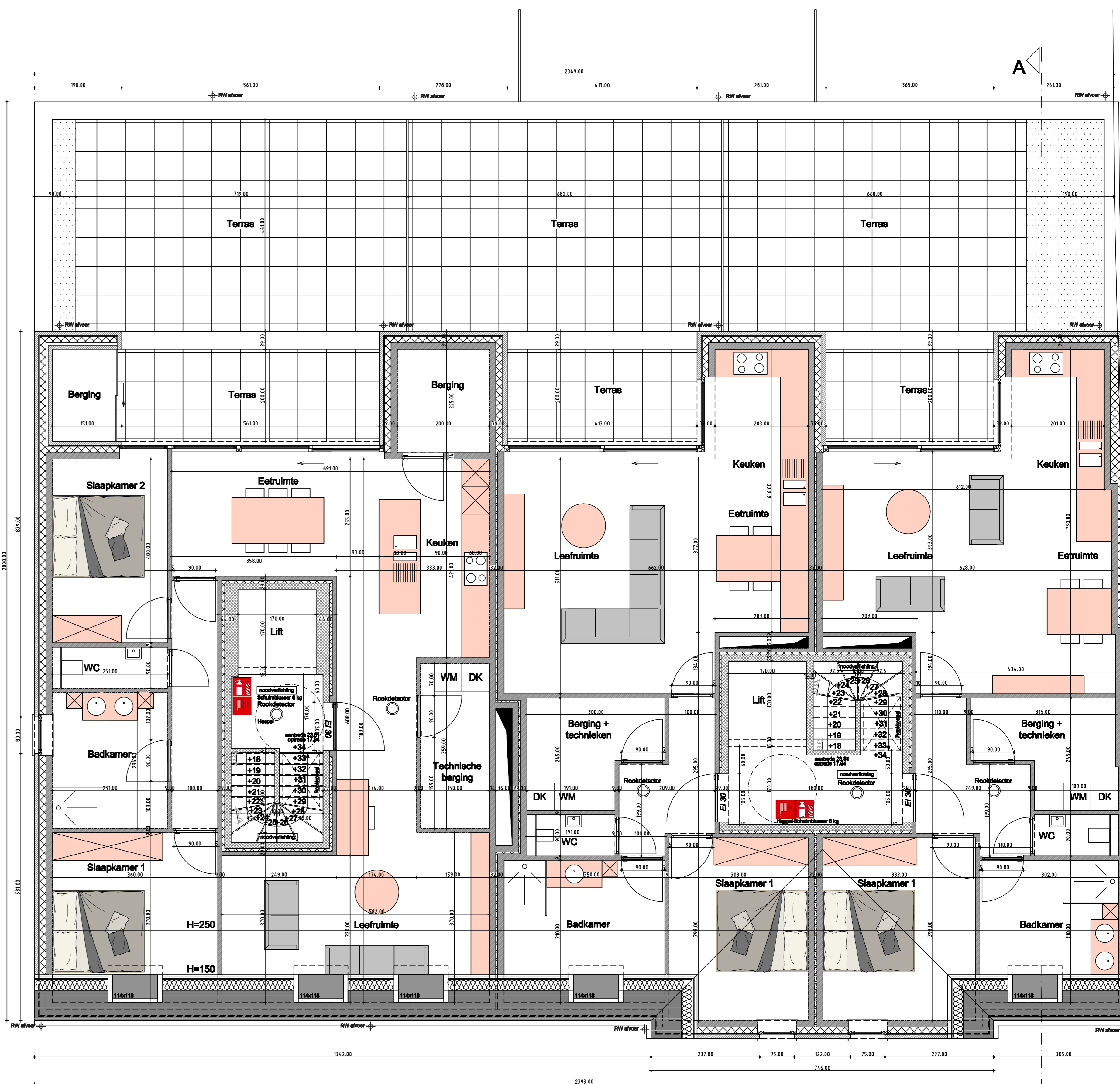
appartement 7 : 2 slaapkamer appartement verdieping +2 schaal 1/50 opp. 124.36 m2 terras opp. 11.20 m2
