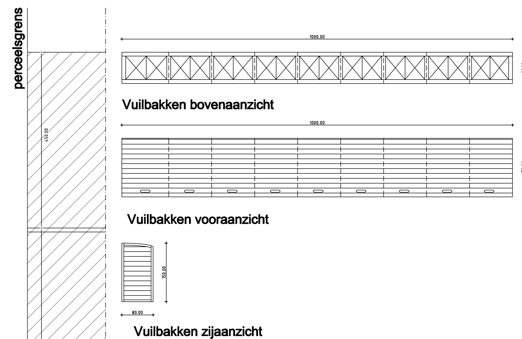
Vuilbakken zijaanzicht
